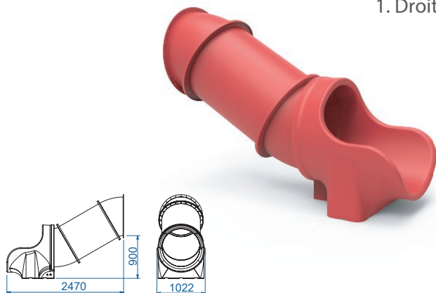
1. Straight 90 1. Droit 90
