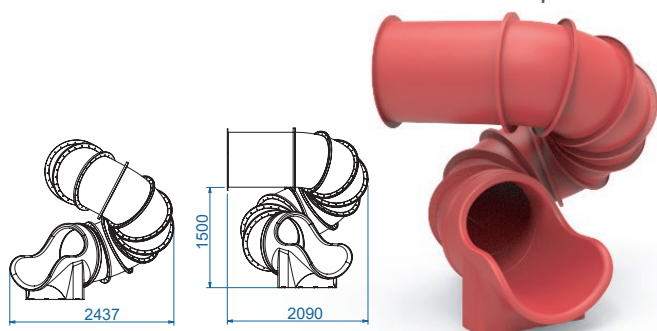
7. Spiral 150 7. Spirale 150
